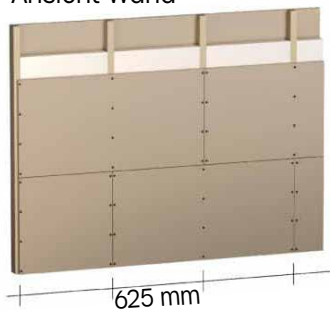
Ansicht Wand
