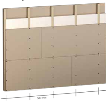
Plaatsing wand
