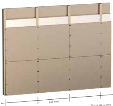
Ansicht Wand
